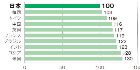
図1 転炉鋼の一次エネルギー原単位推定結果 (2015年、日本を100とした時)
