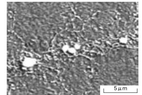
写真5 旧オーステナイト粒界に析出した炭化物(WC)
