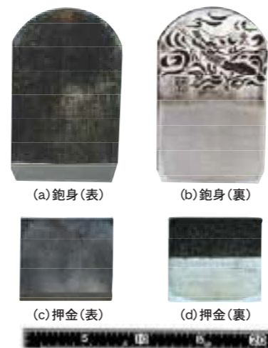
写真2 平鉋の鉋身と押金
