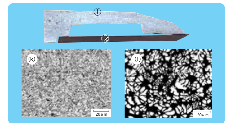
写真8 替刃式の鉋身と押金のマクロ組織及び光学顕微鏡組織 (k)鉋身(l)押金
