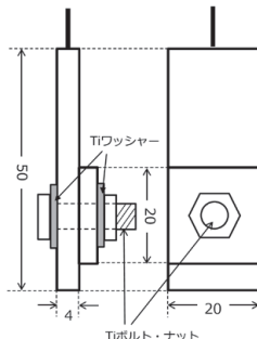
図3 試験片例
